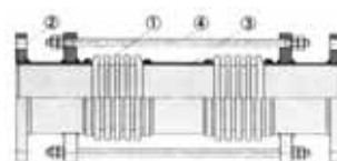
DU800 橫向伸縮接頭
