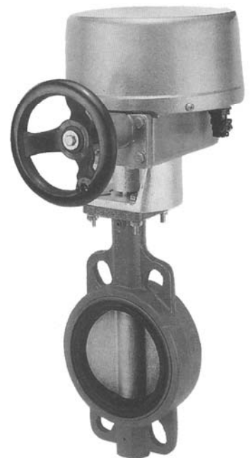
電動式蝶閥
